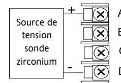
Module d'entrée analogique
