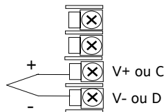
PV fixe (ou module d'entrée analogique)
