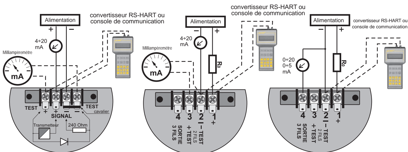
Version : APC-2000ALE avec signal de sortie 4...20mA
